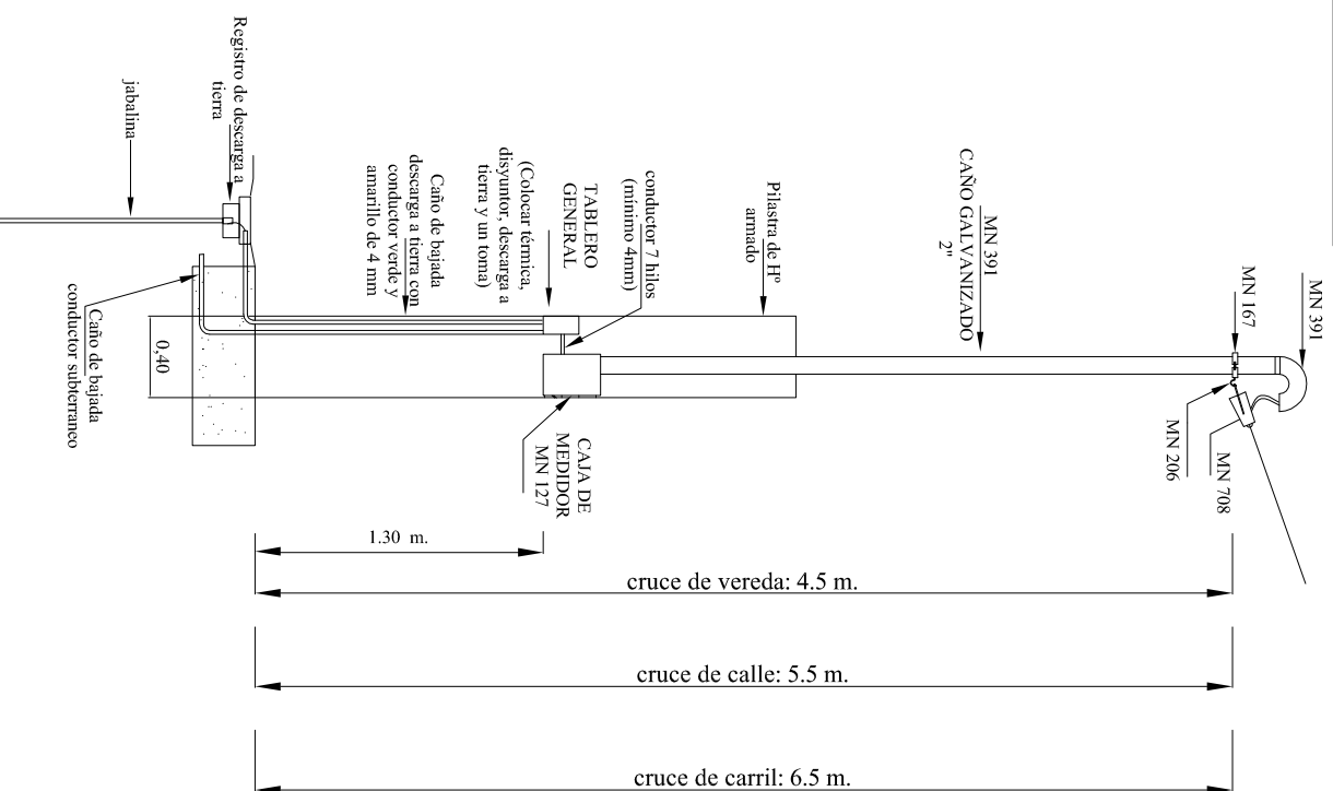
B) Acometida en pilastro
